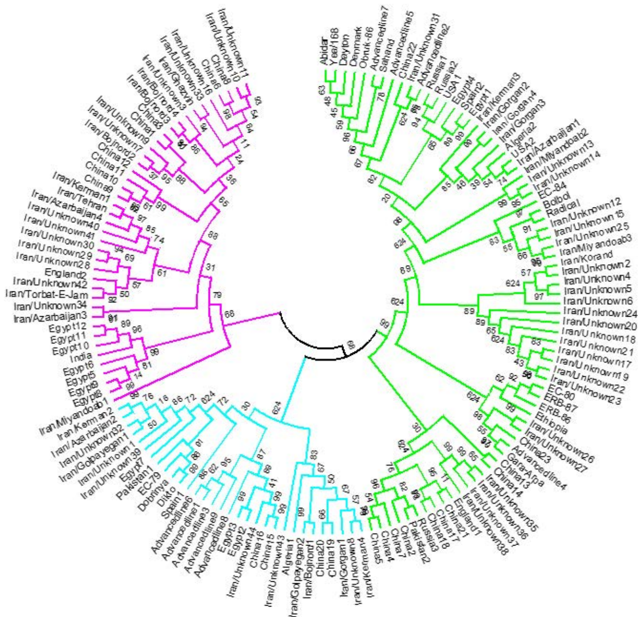
شکل ۲- گروه‌بندی ژنوتیپ‌های جو مورد مطالعه بر اساس داده‌های نشانگرهای ریزماهواره و با استفاده از الگوریتم
