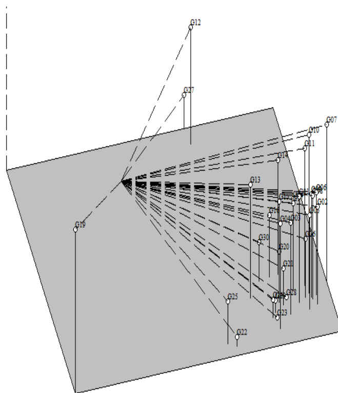
شکل ۵- نمودار پراکنش سه بعدی ژنوتیپ‌های سنجد بر اساس تجزیه به محوره‌های اصلی با استفاده از نشانگر AFLP Figure 5. Trimensonal scatter plot of Russian olive genotypes based on principle co-ordinate analysis using AFLP markers
