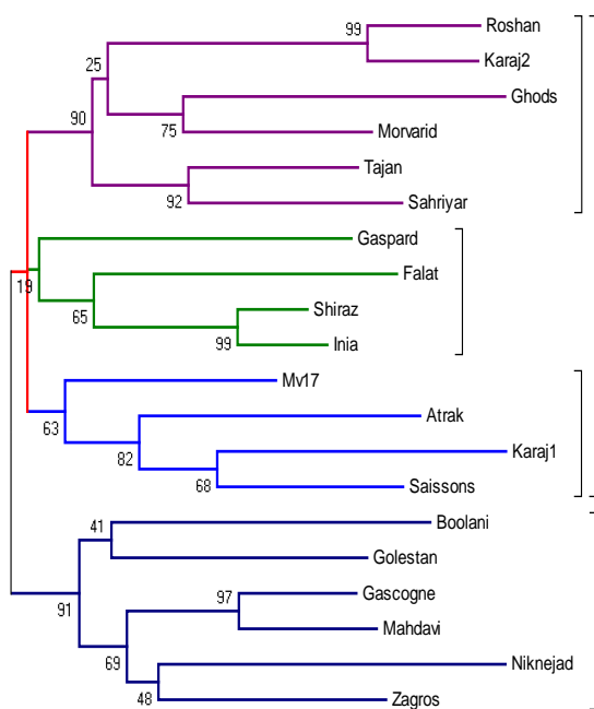
شکل ۲- گروه‌بندی ارقام گندم نان براساس داده‌های نشانگرهای RGA با استفاده از الگوریتم Neighbor
