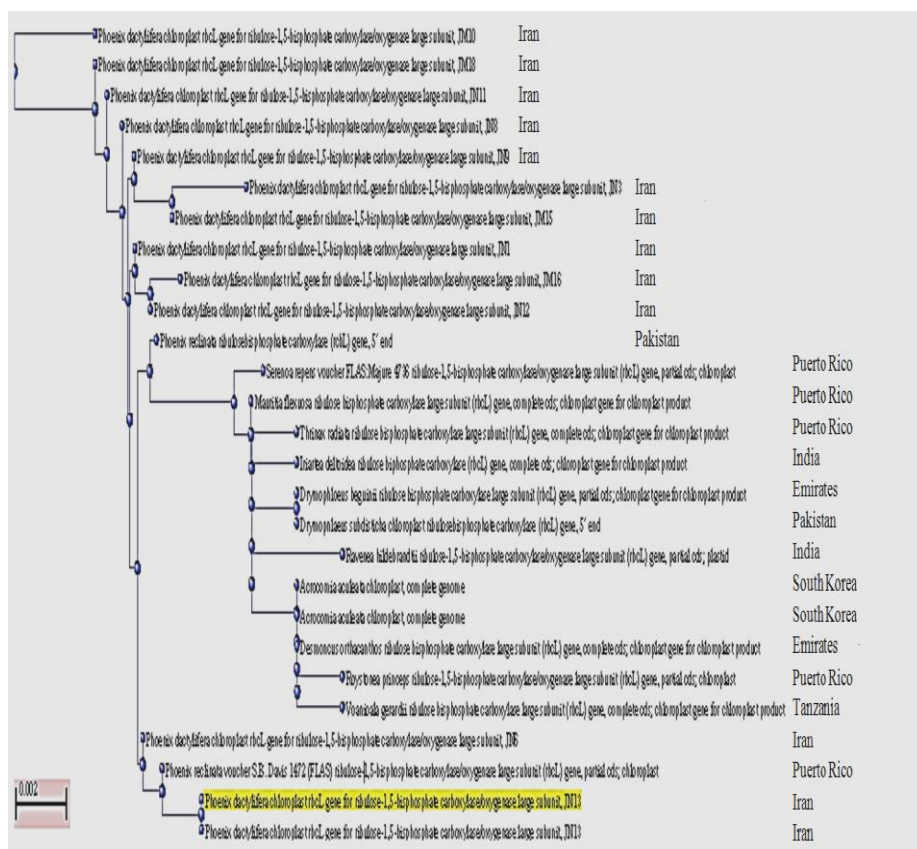
شکل ۶- آنالیز خوشه‌ای ۱۵ رقم خرمای مورد مطالعه و ژنوتیپ‌های نخل خرمای برخی کشورهای دیگر بر اساس ناحیه توالی‌یابی شده ژن rbcL Figure 6. Cluster analysis of 15 studied date palm genotypes and date palm genotypes from other countries, based on the rbcL sequenced region available in NCBI database
