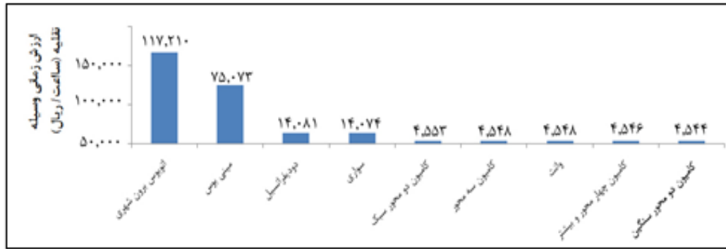
شکل ۷. نمودار نزولی ارزش زمانی وسیله نقلیه حاصل از نتایج نرم افزار RUCKS
