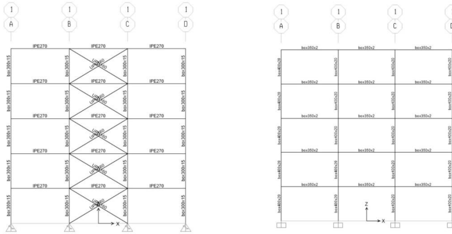
شکل ۶. مدلسازی قاب ۵ طبقه
