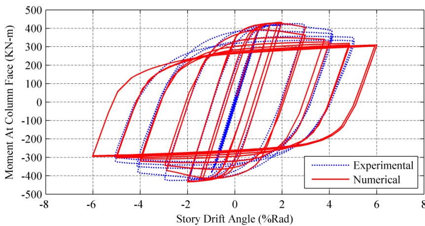
شکل ۷. صحت سنجی با نمونه‌ی آزمایشگاهی مرجع [۶]
