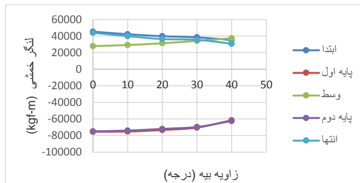
شکل ۱۵. نمودار لنگر خمشی M_3 عرشه بر حسب زاویه بیه در فواصل مختلف از ابتدای دهانه
